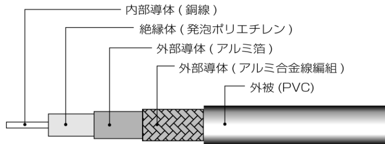
S-4C-FB 同軸ケーブル概要
